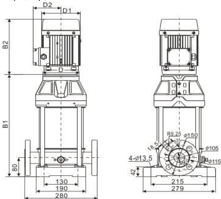
Размеры, мм
