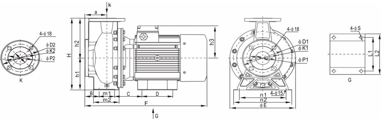
Габаритный чертёж
