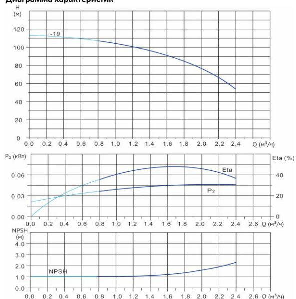
Диаграмма характеристик
