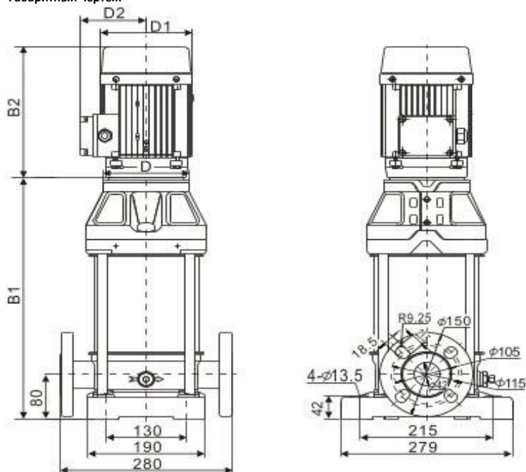
Размеры, мм
