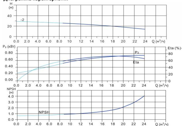
Диаграмма характеристик
