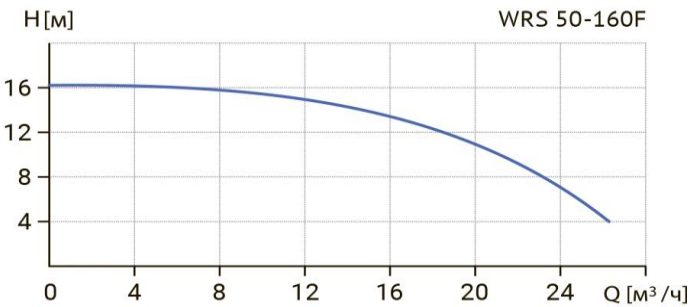
Диаграмма характеристик
