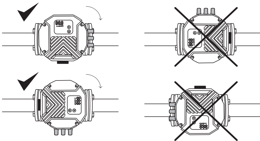
Рисунок 3. Допустимые положения блока управления отмечены
