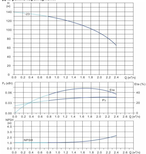
Диаграмма характеристик
