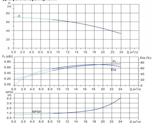
Диаграмма характеристик
