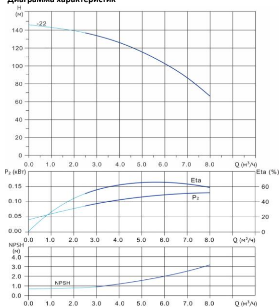
Диаграмма характеристик
