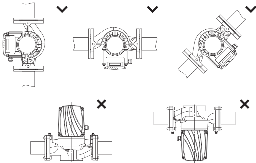
Рис. 1 Допустимые положения насоса
