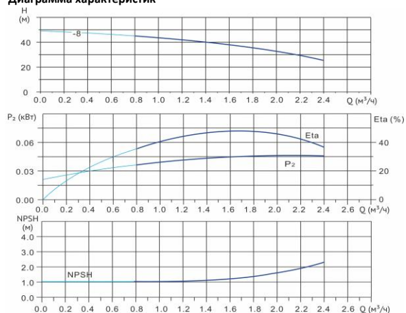
Диаграмма характеристик
