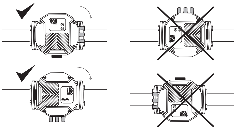
Рисунок 3. Допустимые положения блока управления
