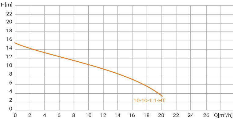
Диаграмма характеристик
